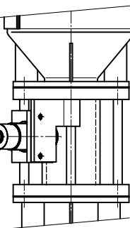
Auxiliary packing 補助パッキン Sensor periphery センサ外周部
