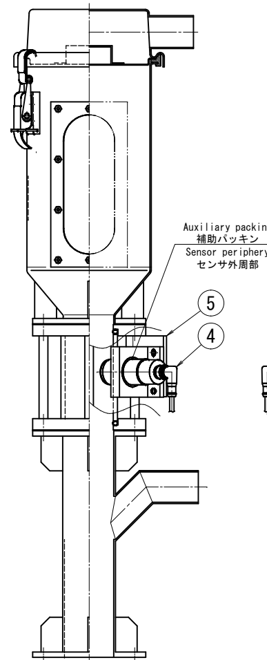
Standard dwg. 標準図
